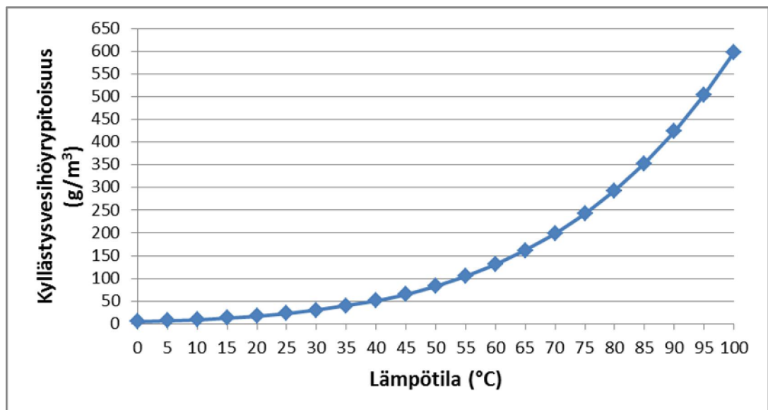
Kuva 3-1. Ilman kylästysvesihöyrypitoisuus lämpötilan funktiona.
