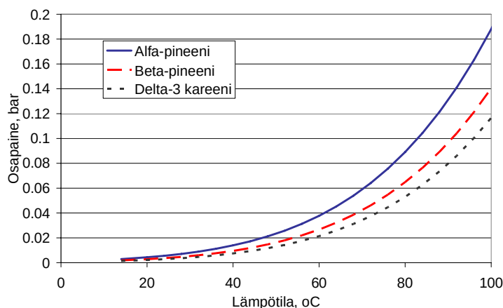
Kuva 12-1. Tärpätin komponenttien höyryn osapaineita, Drew et al., 1971
