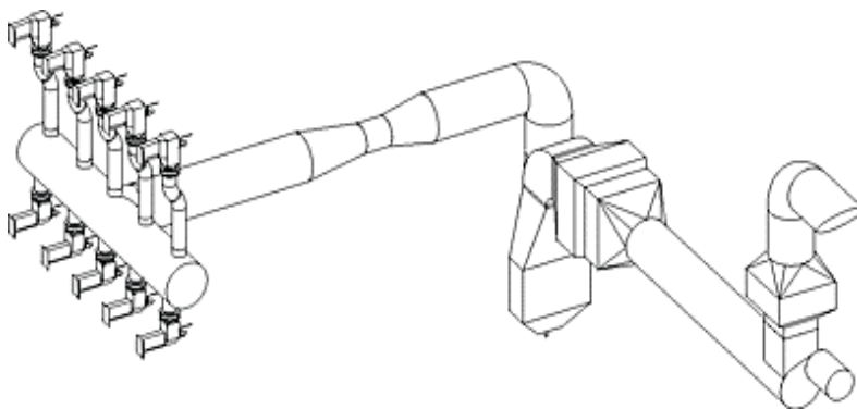
Kuva 5-15-1. Esimerkki laimeiden hajukaasujen kanavistosta
