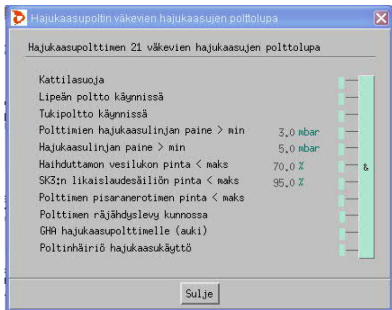
Kuva 7-27-2. Esimerkki erään tehtaan väkevien hajukaasujen polttoehdoista
