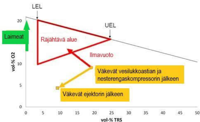
Kuva 2-2. Räjähdykskolmio
