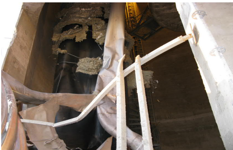
Kuva 15-13-1. Kuva sisäpiipusta räjähdysen jälkeen
