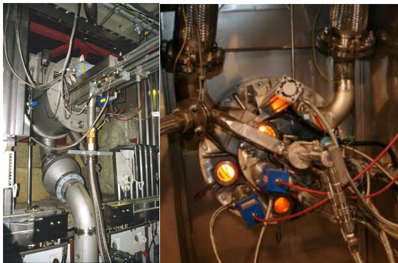
Kuva 2-12-1. Väkevien hajukaasujen poltin
