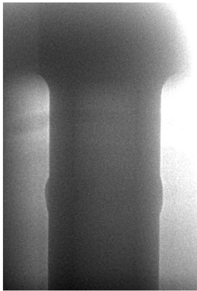
Röntgenkuva suutinputkesta
