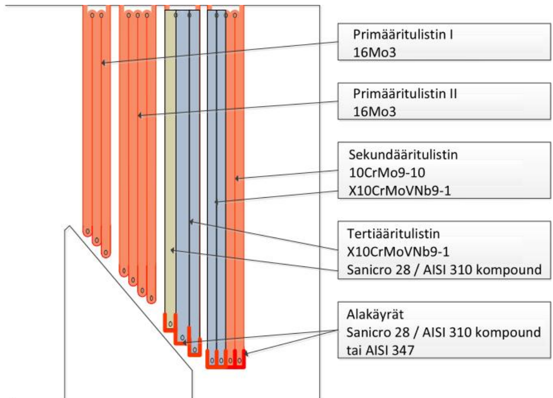
Kuva 1-4. Esimerkki paremman lujuuden / suuremman korroosiovaran tulistinmateriaaleista
