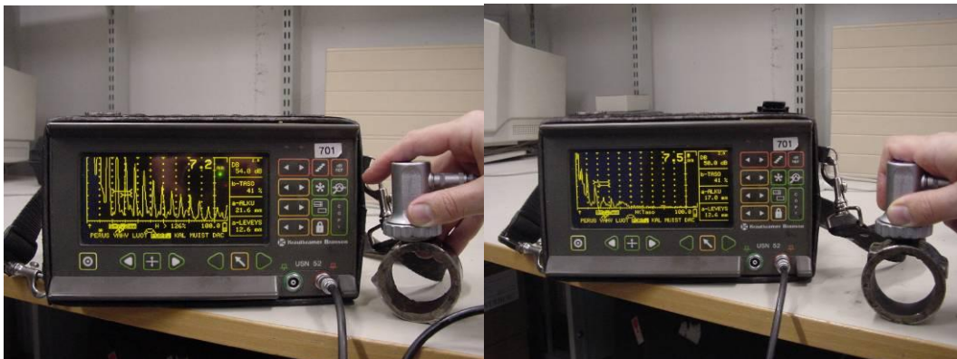
Kuva 4-104-10. A-näytöt ehjästä putkesta ja vetyhyökkäyskohdalta.
