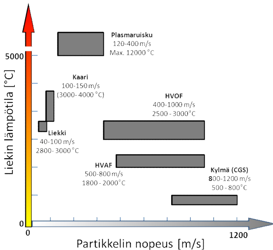
Kuva 2-12-1. Eri prosessien tuottama ruiskutuspartikkelien nopeus ja liekin lämpötila-alue.
