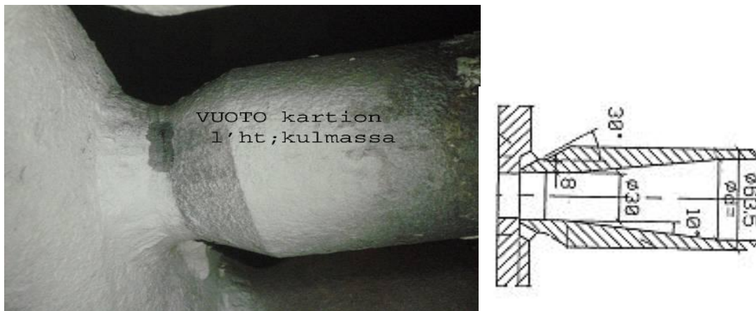
Kuva 4-14-1. Ekonomaiserin jakotukin yhde.
