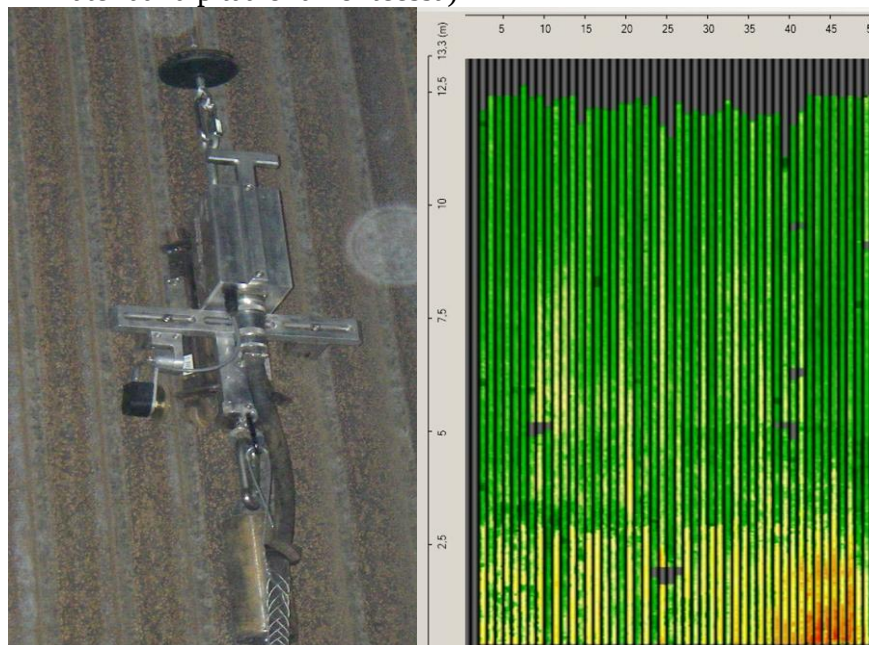
Kuva 4-84-8. T-scan laitteisto kattilan seinällä ja Client ohjelmiston tuottamaa visuaalista paksuusmittaustulosta tarkastuksista.
